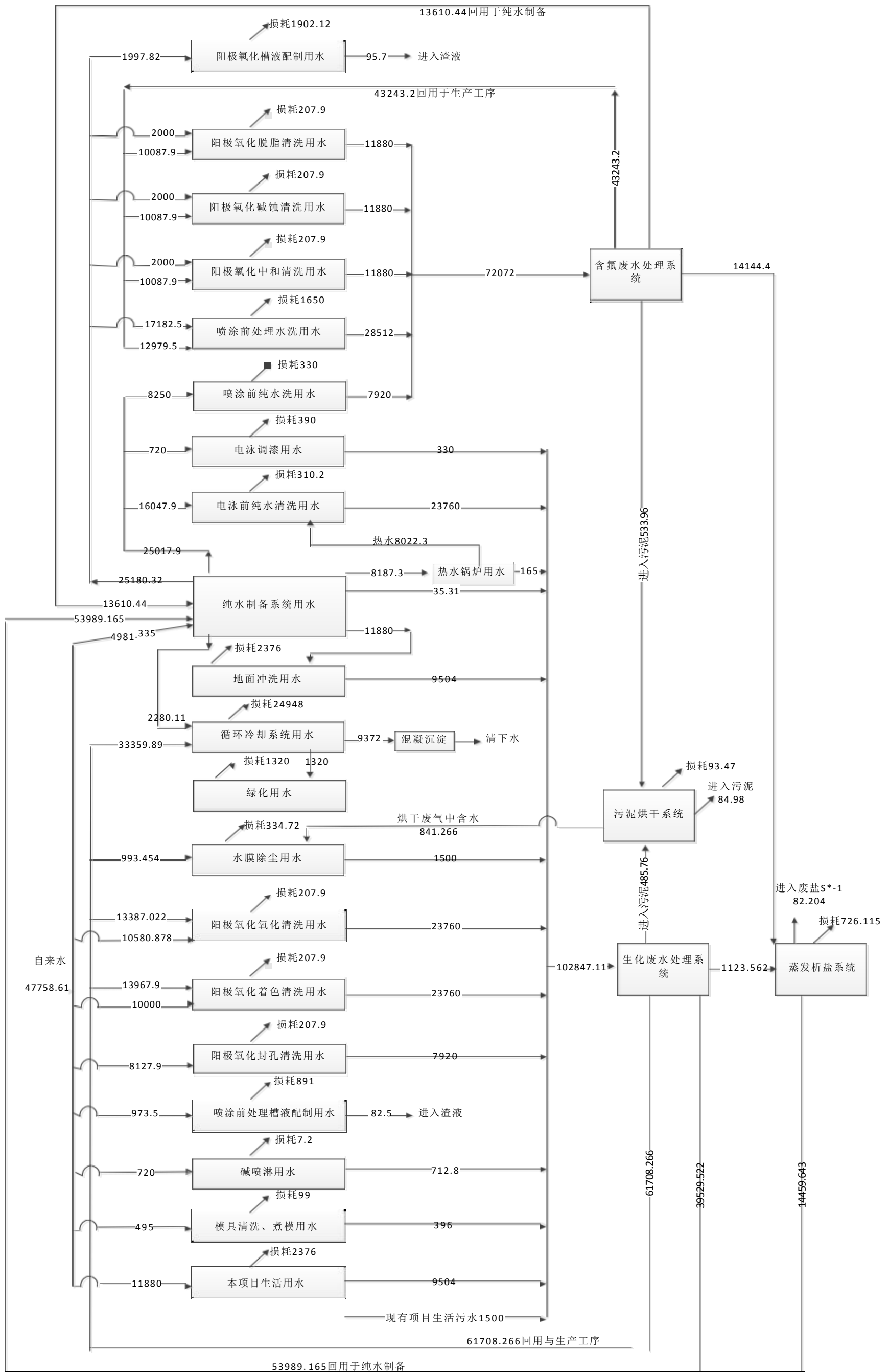
江苏库纳新能源股份有限公司水平衡图
